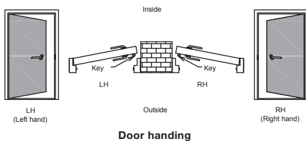
Door handing
