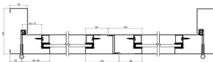
Double Door Section
